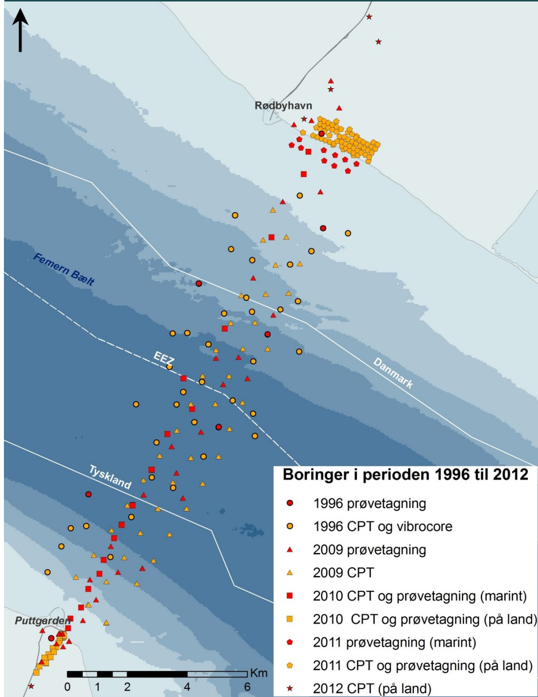
FIGUR 10.5-2 Placeringen af undersøgelsesboringer
