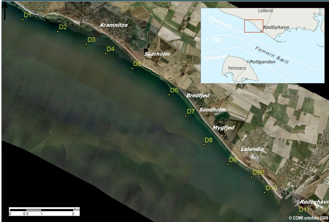
FIGUR 10.1.4-16 Eksempler på modelberegnete kystnære bølgeroser vest for Rødby
