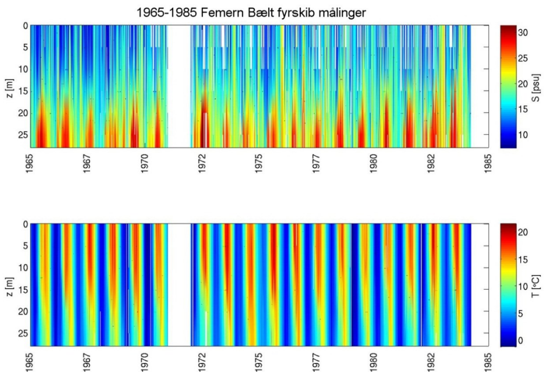
FIGUR 10.1.1-29 Målt salinitet og temperatur ved Femern Bælt fyrskib fra 1965 – 1985 (FEHY 2013b)
