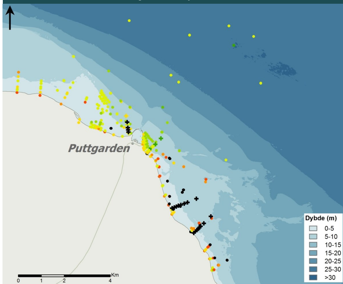
FIGUR 10.1.4-33 Korndiameter d50 langs Fehmarns kyst
