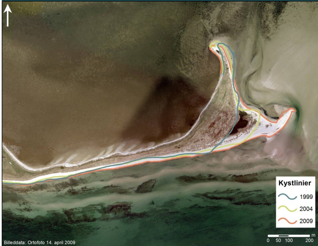
FIGUR 10.1.4-13 Kystlinjeændringer i perioden 1999 - 2009 ved den østligste del af Hyllekrog
