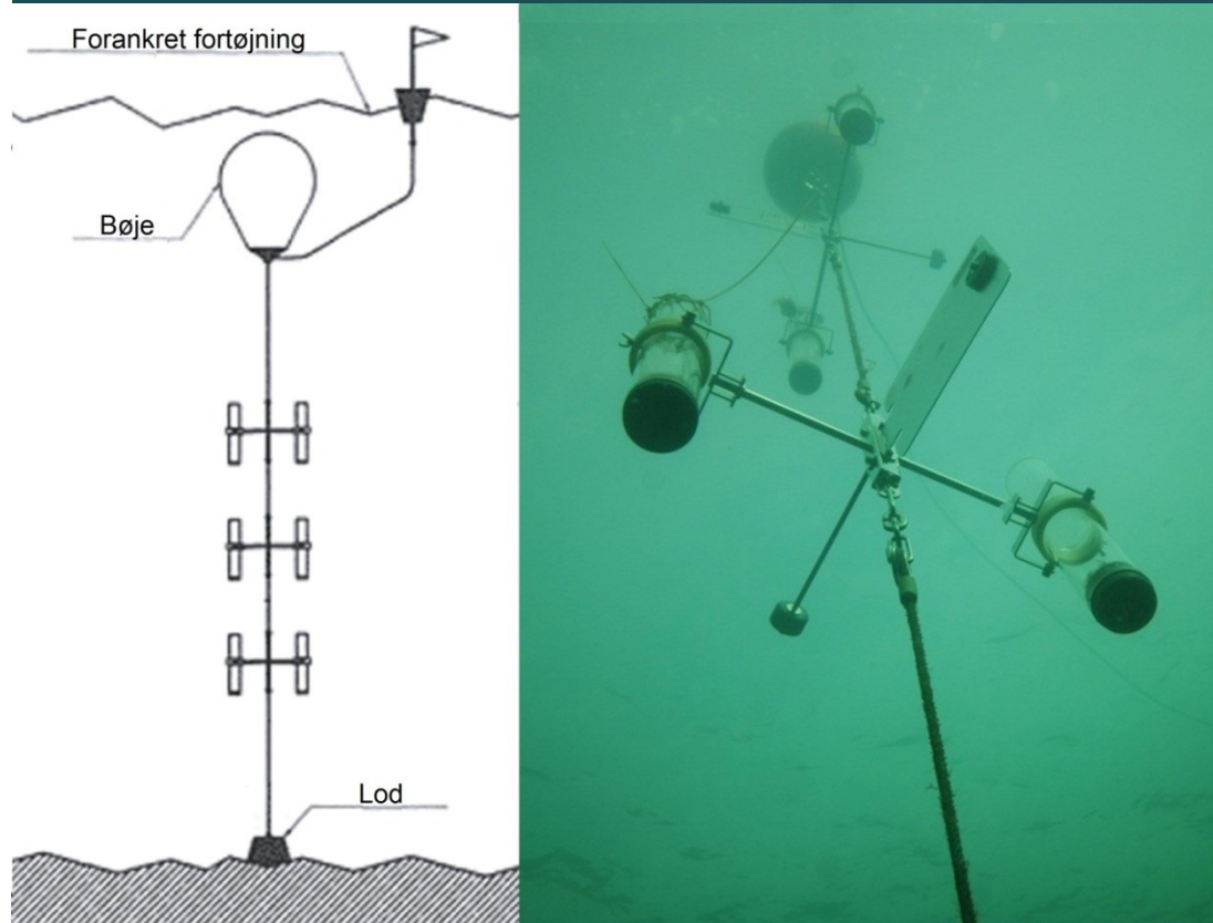
FIGUR 10.1.2-12 Skitse og foto af en sedimentfælde
