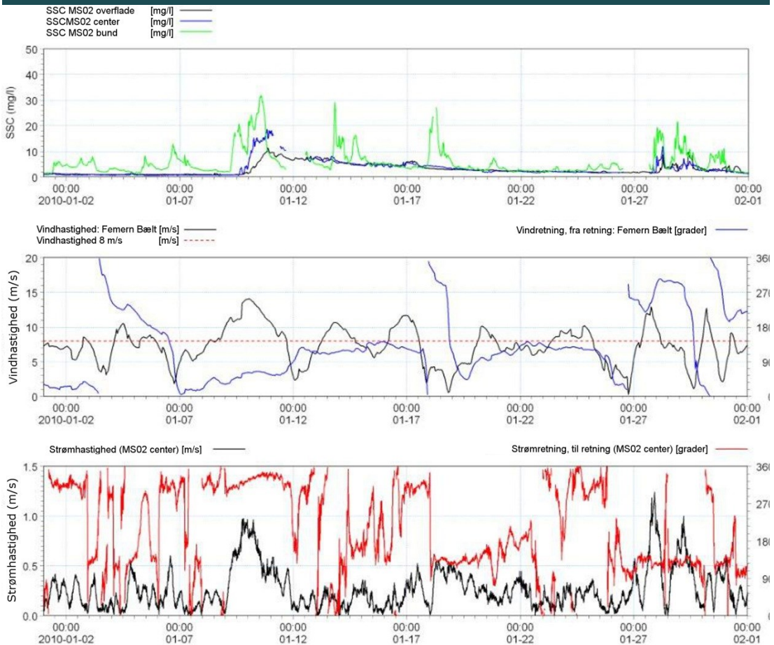
FIGUR 10.1.2-19 Sedimentkoncentrationer, vindhastighed og – retning og målte strømshastigheder og -retninger i midtddybe på station MS02 fra januar 2010
