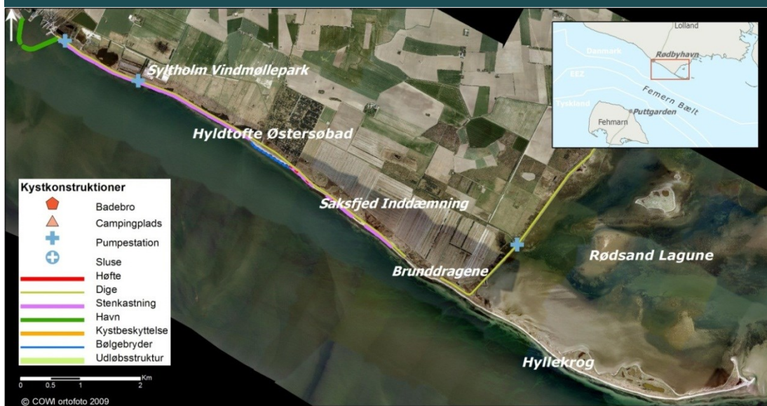
FIGUR 10.1.4-9 Oversigt over kystkonstruktioner mellem Rødbyhavn og Hyllekrog
