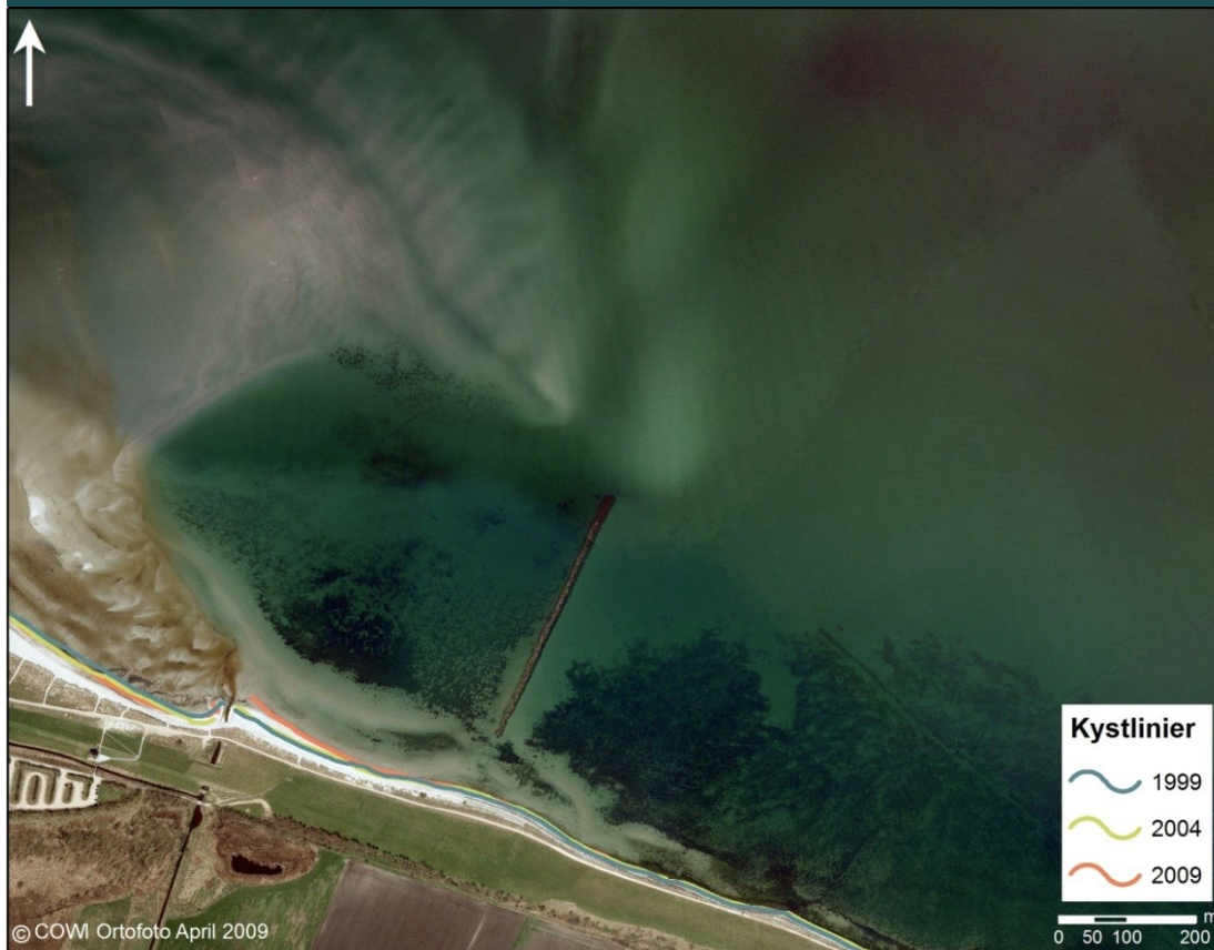
FIGUR 10.1.4-31 Den fritliggende høfde og konstruktionerne ved udløbet mellem Grüner Brink og Puttgarden Havn
