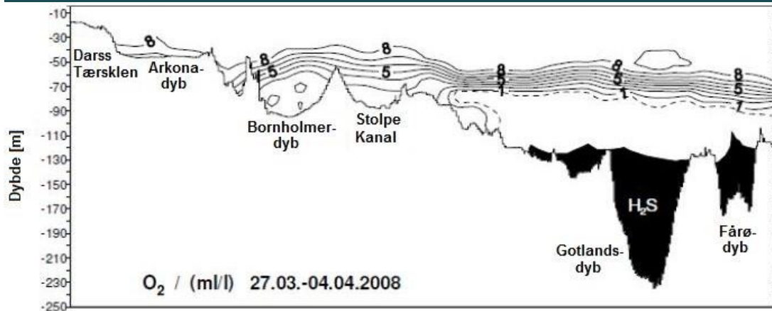
FIGUR 10.1.2-4 Fordeling af ilt og svovlbriente i et transekt fra Darss-tærsklen til Fårø Dyb i den centrale Østersø (fra Nausch et al., 2009)
