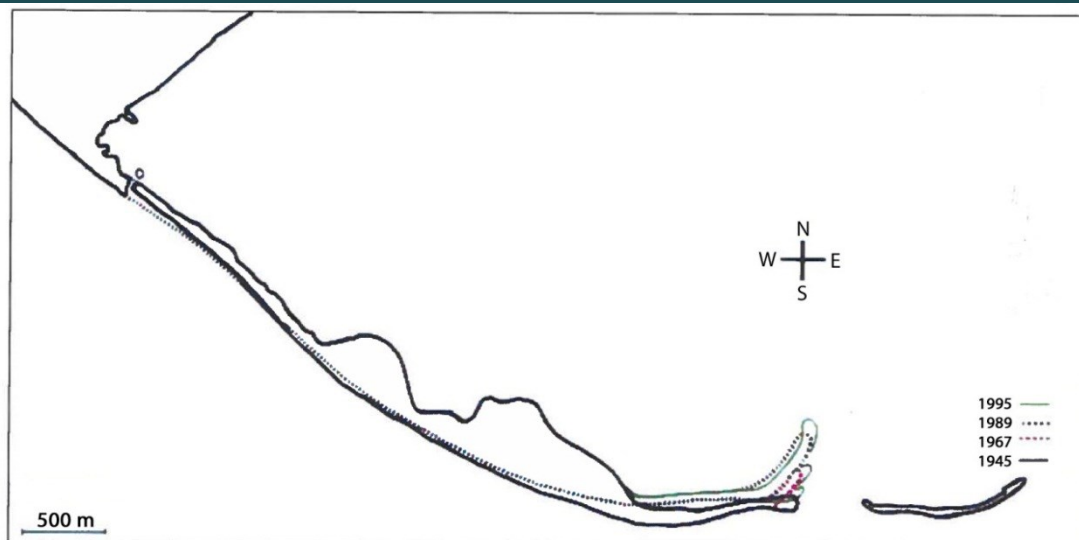
FIGUR 10.1.4-7 Udvikling af Hyllekrog 1945 - 1995 (Jensen 2006)
