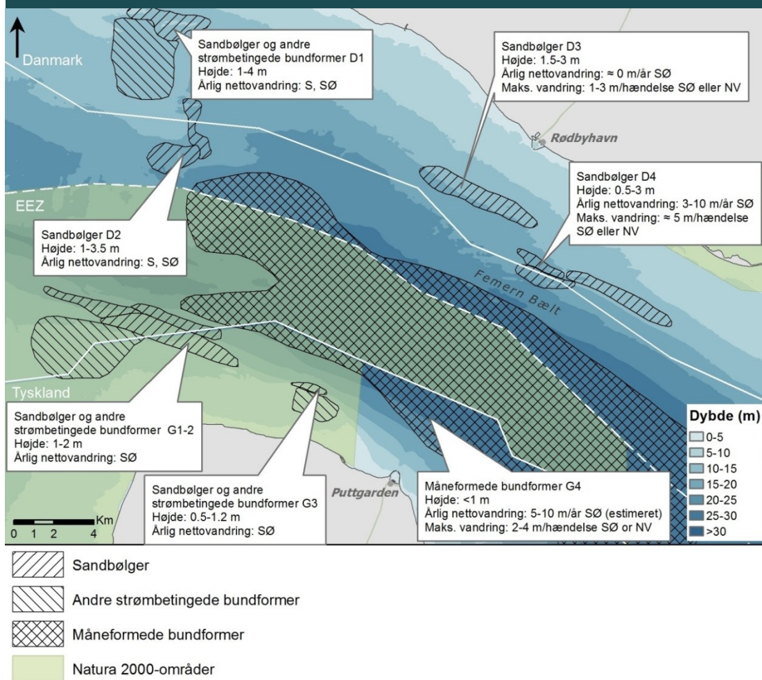
FIGUR 10.1.3-17 Områder med markante bundformer i Femern Bælt
